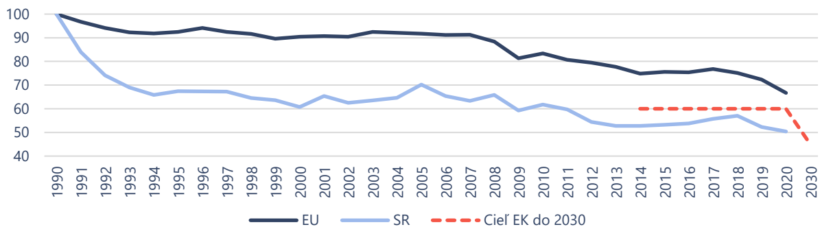
Graf 1: Čisté emisie skleníkových plynov v EÚ a SR v rokoch 1990 – 2020 (index: 1990 = 100)
