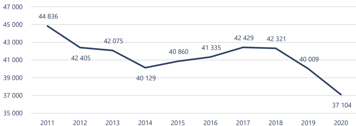
Graf 2: Celkové emisie skleníkových plynov a znečisťujúcich látok na Slovensku (v tis. ton)
